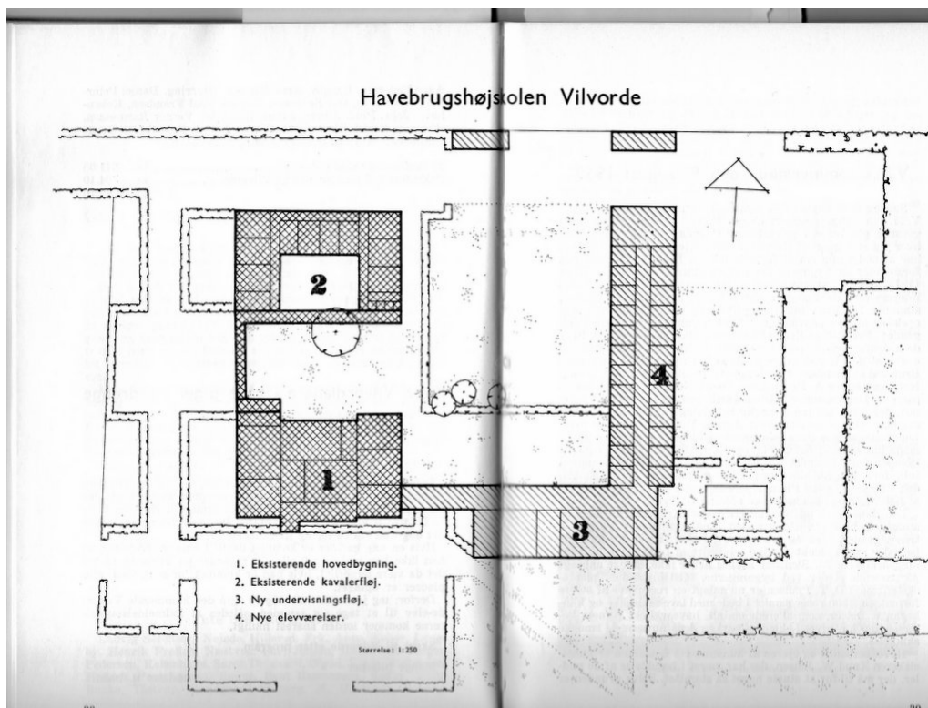
Figur 21. Grundplan efter udvidelsen i 1961
